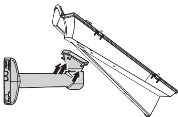
Fig. 6 Fissaggio su supporto con passaggio interno dei cavi.
