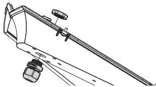
Fig. 2 Supporto per passaggio esterno dei cavi.
