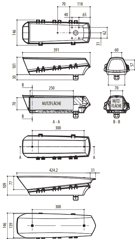
Abb. 14 PUNTO Hi-PoE.
