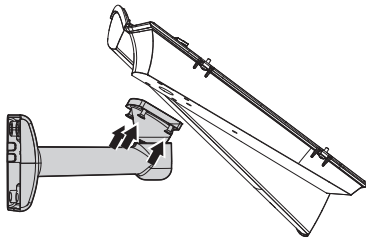
Abb. 6 Befestigung auf der Halterung mit interner Kabeldurchführung
