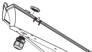
Abb. 2 Halterung mit externer Kabelführung.
